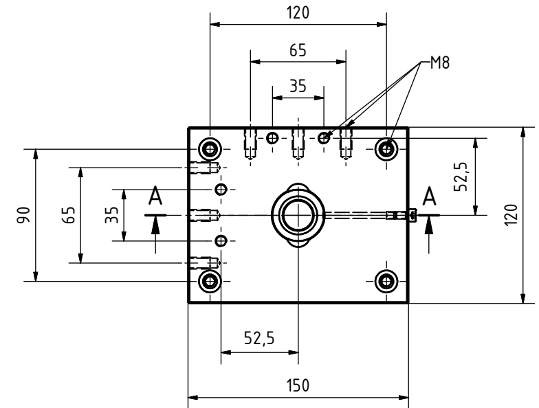
( 1 : 2 ) Adapterstück
