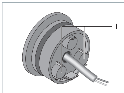
Fig. 6: Position von Trägerprofil und Nasen.
