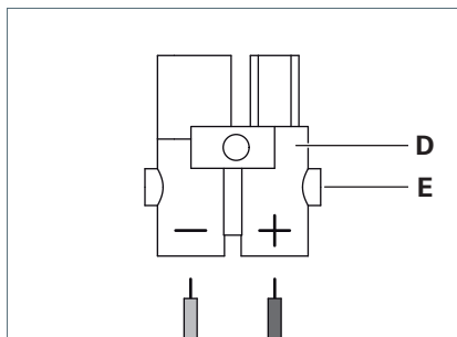
Fig. 4: Steckerbelegung.
