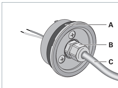
Fig. 3: Luminaire RL70.
