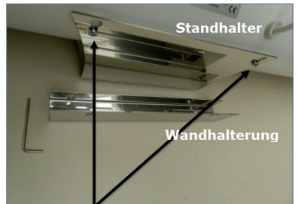
Fig. 5: Schrauben lösen.
